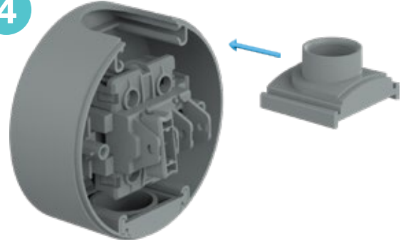
Conta yuvasına boru contasını yerleştirin
